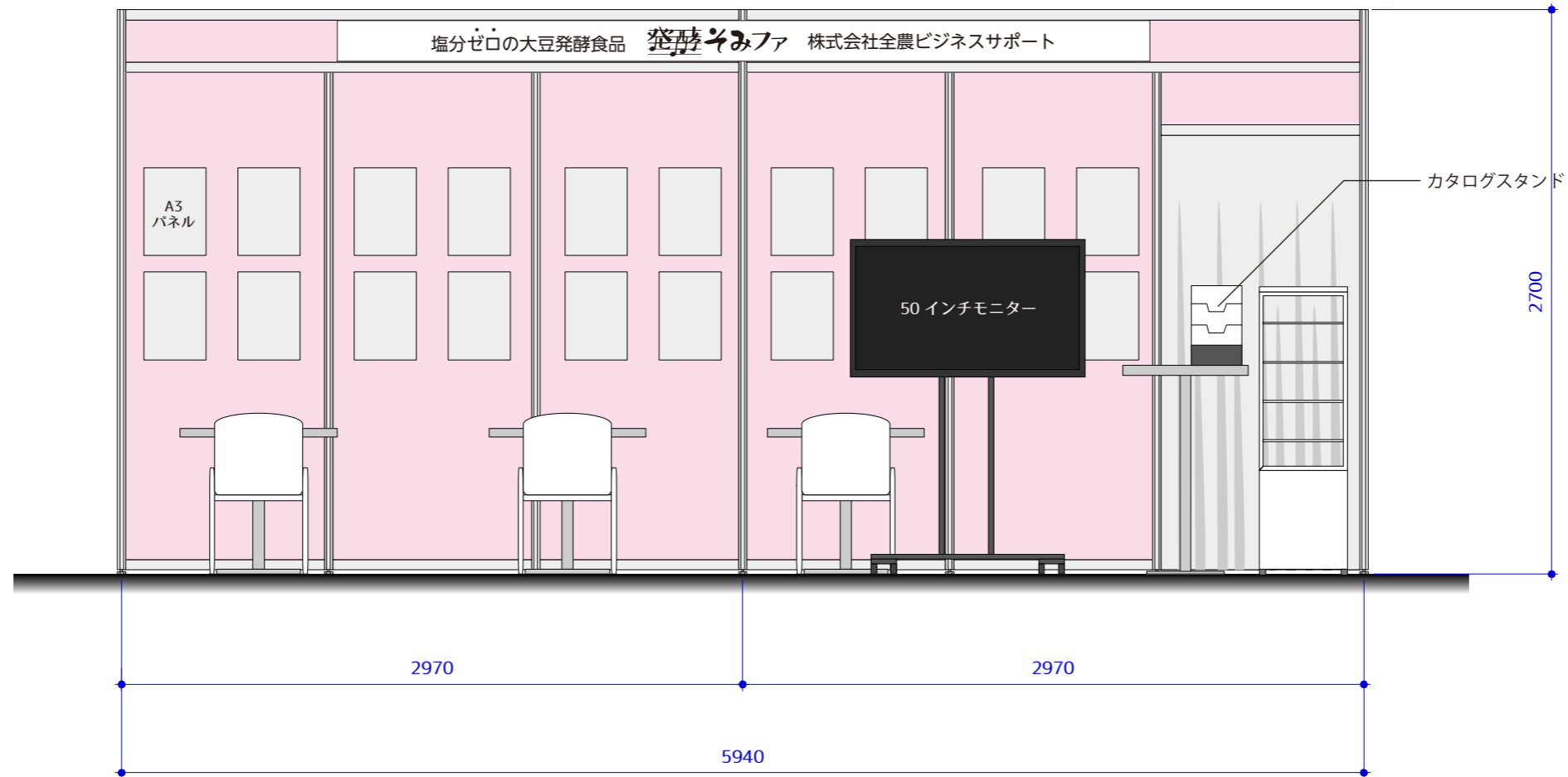
【A- 立面図】
